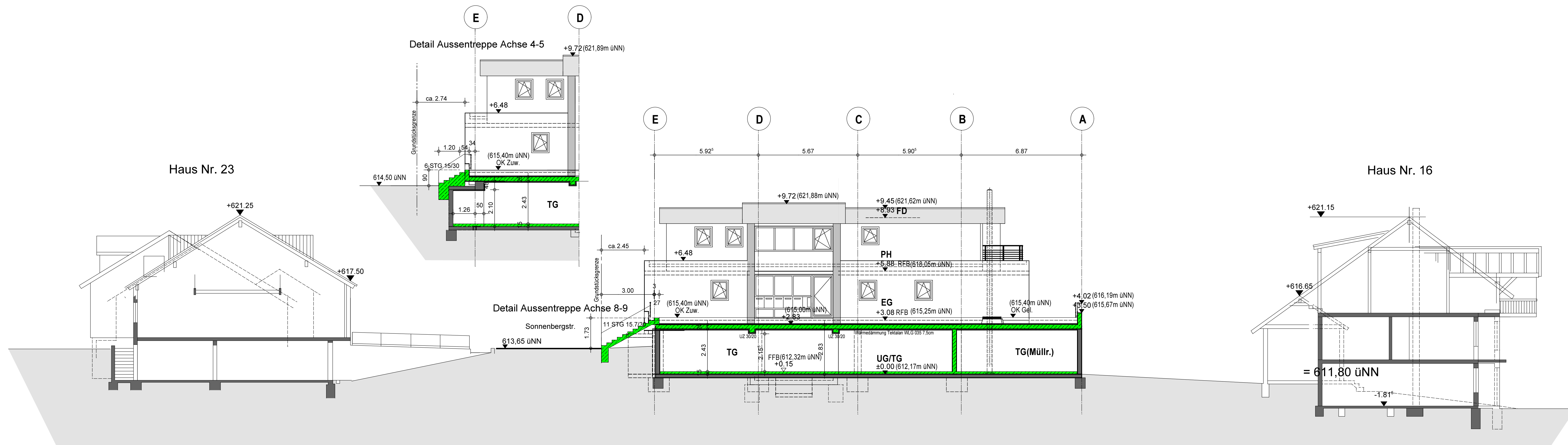
QUERSCHNITT B-B
