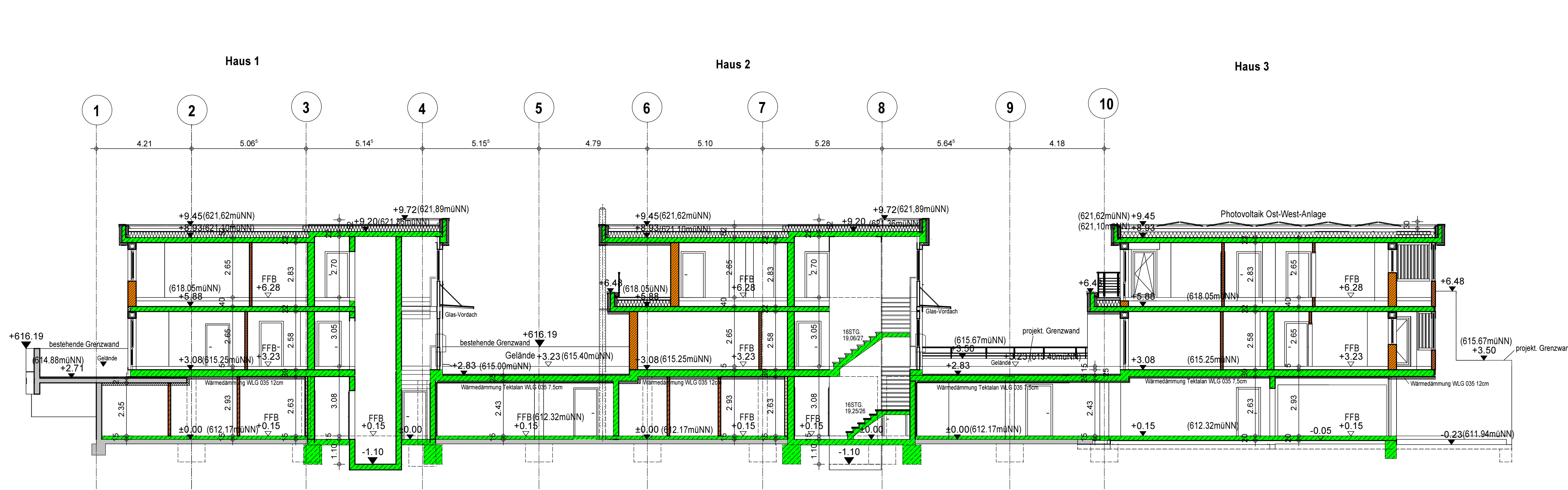
LÄNGSSCHNITT A-A
